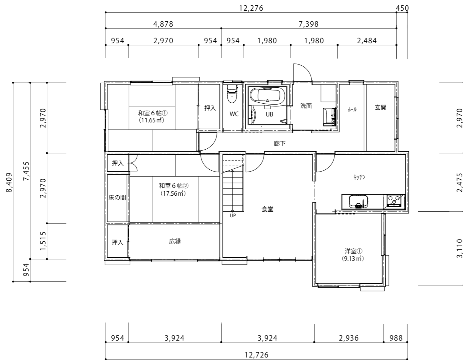
1階平面図
